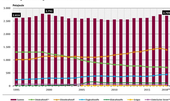
Entwicklung des Endenergieverbrauchs nach Kraftstoffarten
